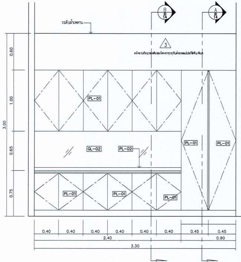
B2 ID-14 รูปด้านหน้า B-2 มาตราส่วน 1: 25
