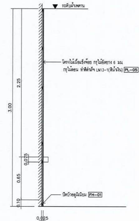
B1 ID-12 รูปตัดที่ B-B มาตราส่วน 1: 25
