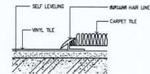
แบบขยาย 1:2 TYP.FLOOR
