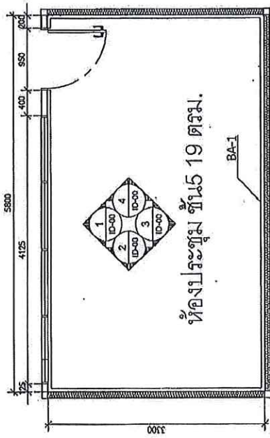
PLAN SCALE 1 : 50
