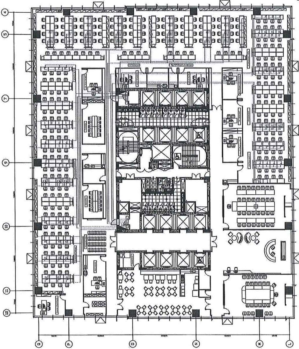
แปลนระบบปลั๊กไฟฟ้า ชั้น 5
