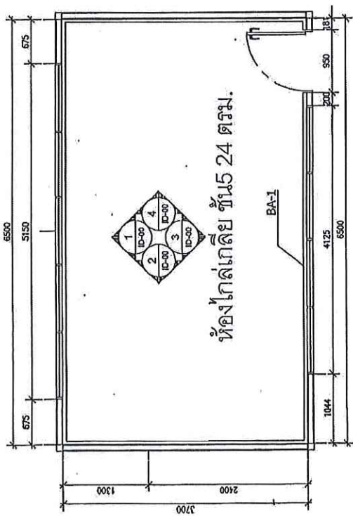
PLAN SCALE 1 : 50
