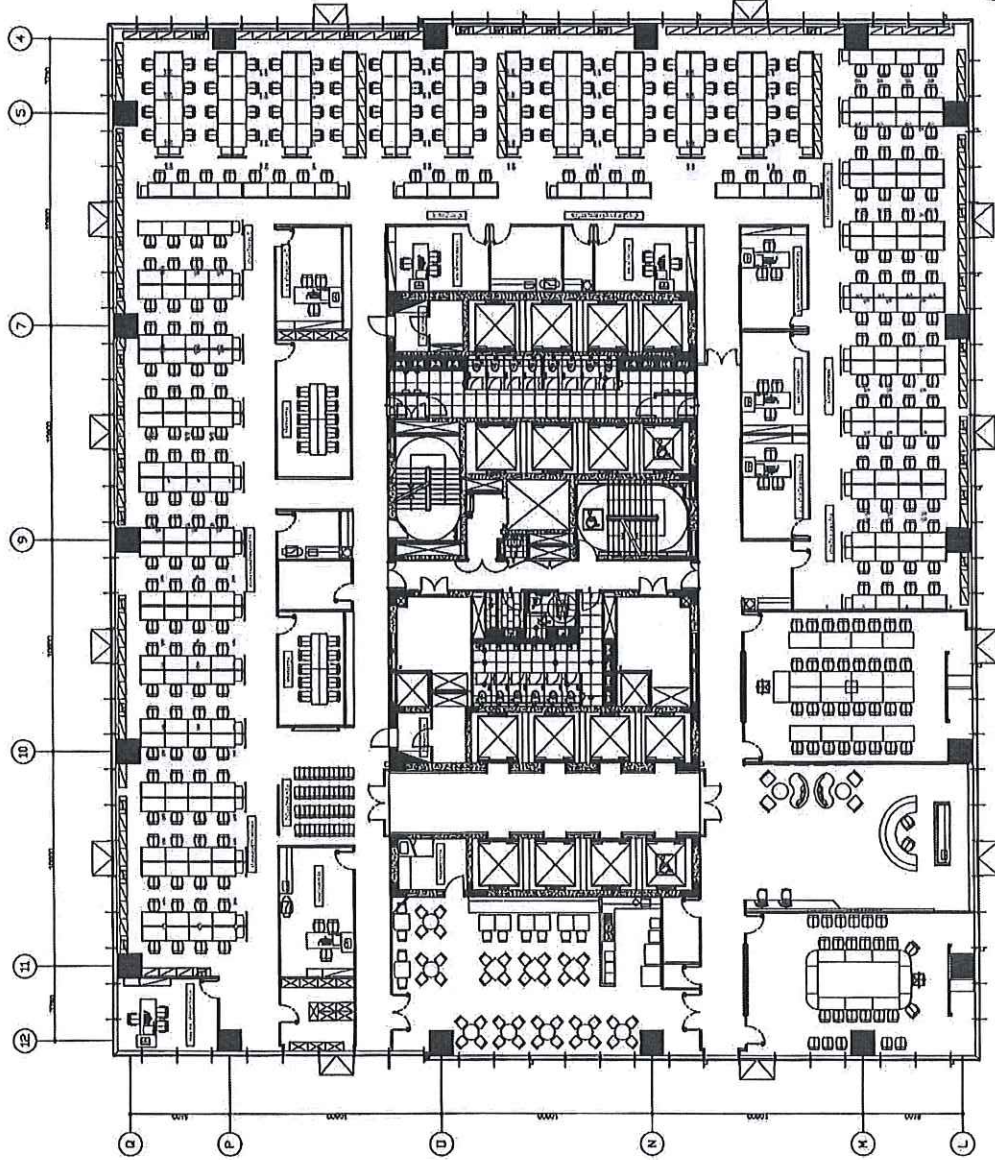
แปลนระบบปลั๊กไฟ ชั้น 5
